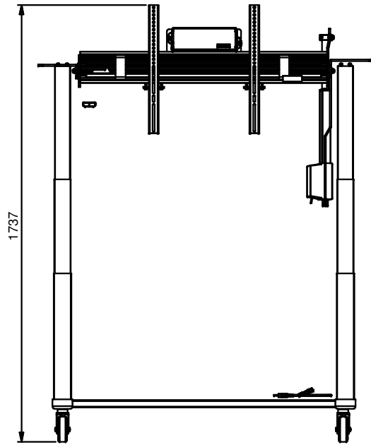
UP VERTICAL 1 : 15
