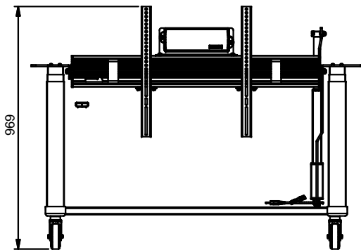
DOWN VERTICAL 1 : 15
