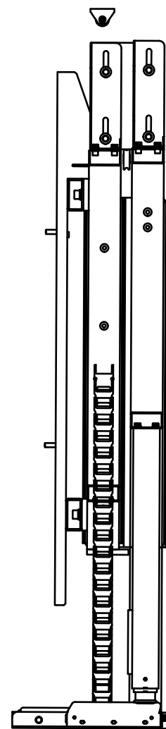
Section A-A ( 1 : 10 )
