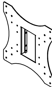
VESA 400
