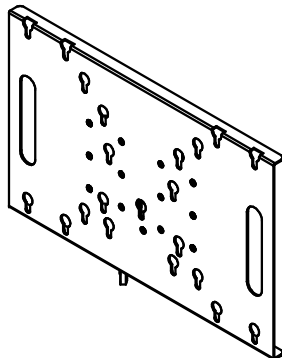
MULTI VESA 1 : 10
